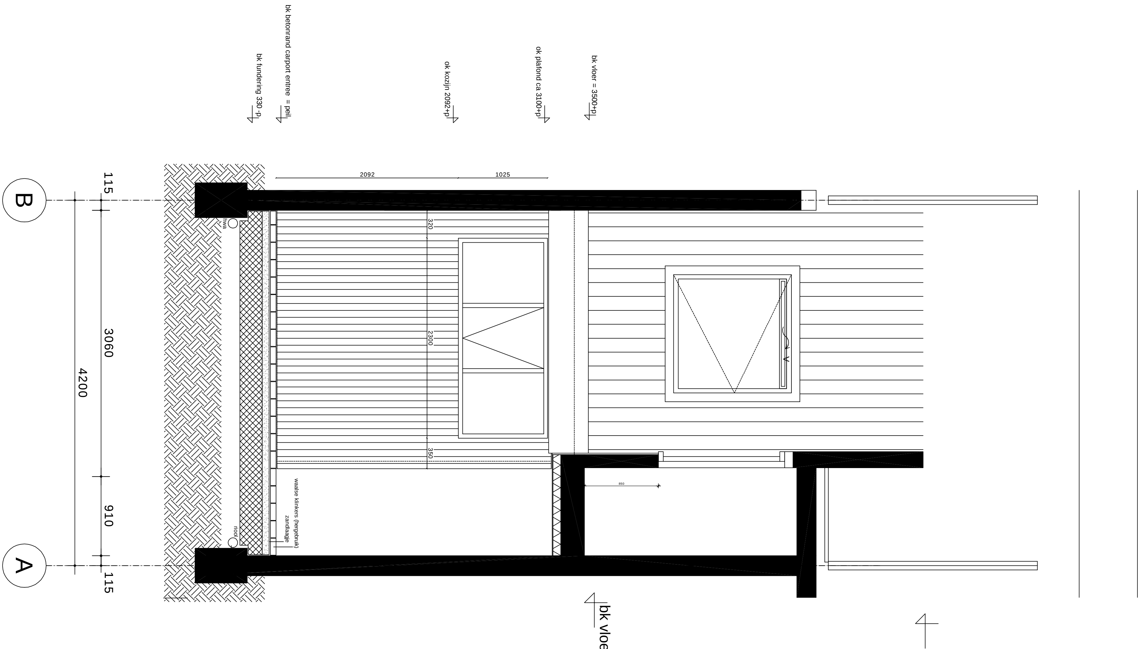
doorsnede B-B'
