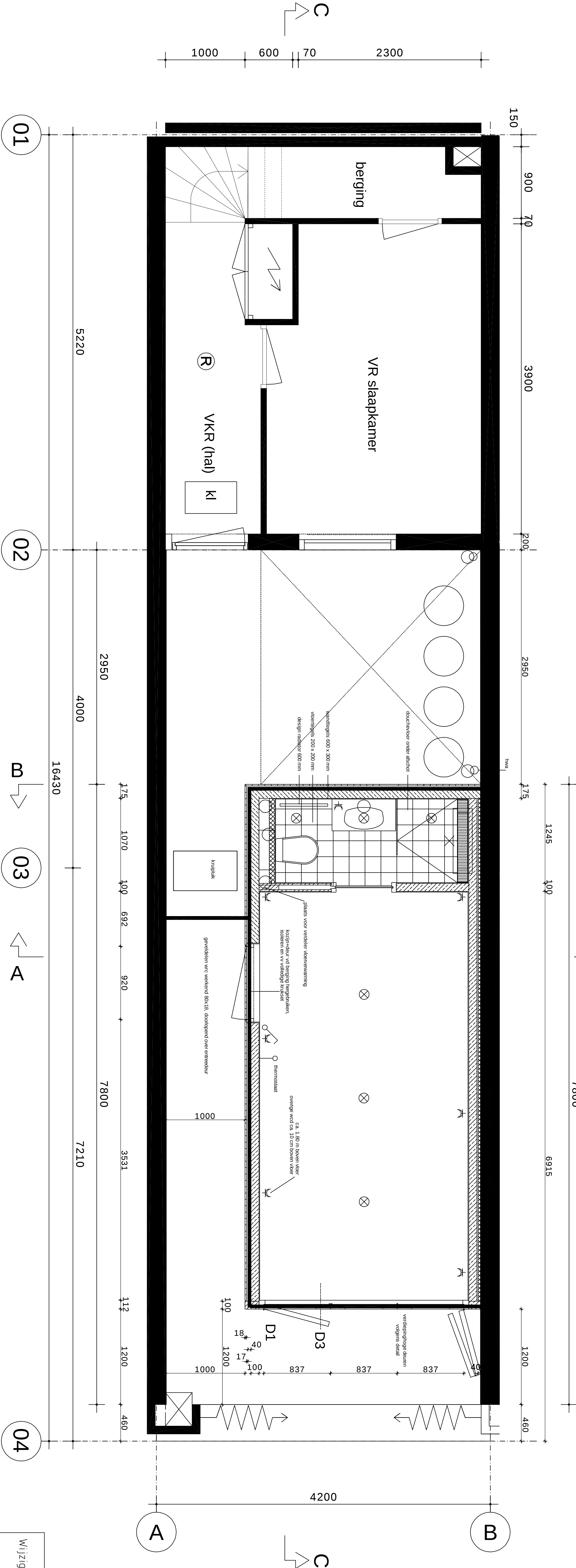
begane grond
